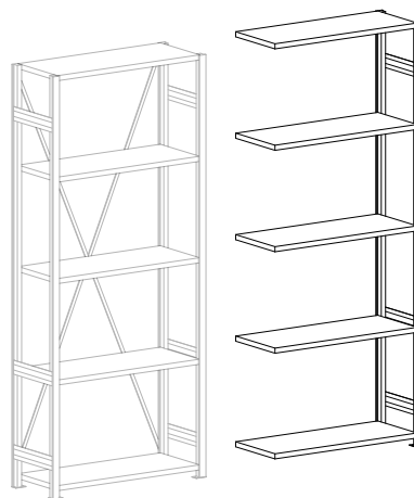
Anbaufeld Arthuro: Ausgestattet mit 1 Regalständer, 2 Metallfüßen, 5 glatte, verzinkte Fachböden inkl. Fachbodenträger, ohne Bodenbefestigung
